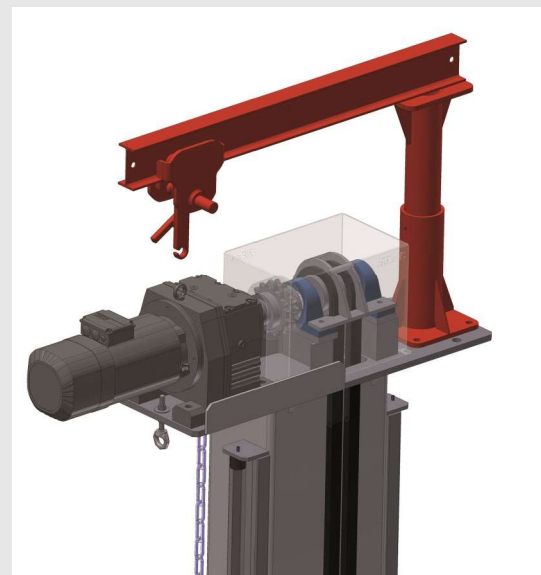
ABG Galgen schwenkbar für Wartung / Reparatur ABG gallow swivel-mounted for service / maintenance
