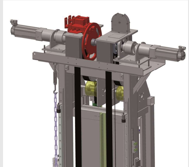
ABS Sicherheitsabsteckung Antriebswelle Lochscheibe ABS safety stacking unit drive shaft indexing disc
