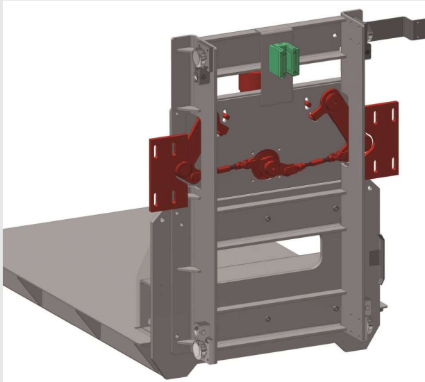
ASB.E Positionsabsteckung elektromechanisch ASB.E position fixation electro mechanical
