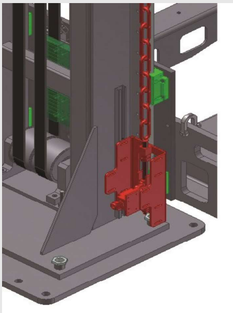
AWK Wartungskette mit Endschalter AWK maintenance chain with limit switch
