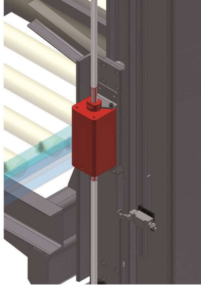
ASB Absturzsicherung Bremse ASB fall protection device brake
