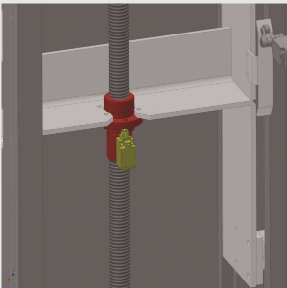
SFM Spindel mit Sicherheitsfangmutter SFM spindle with safety nut
