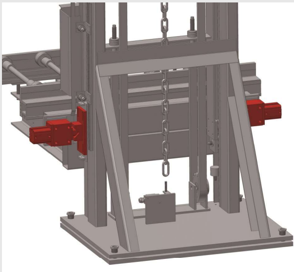
ASB.P Positionsabsteckung prisma pneumatisch ASB.P position fixation prisma pneumatic
