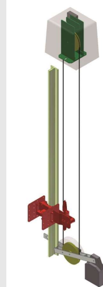
AVS Absturzsicherung mit Wandler Bremse AVS fall protection device with transducer brake
