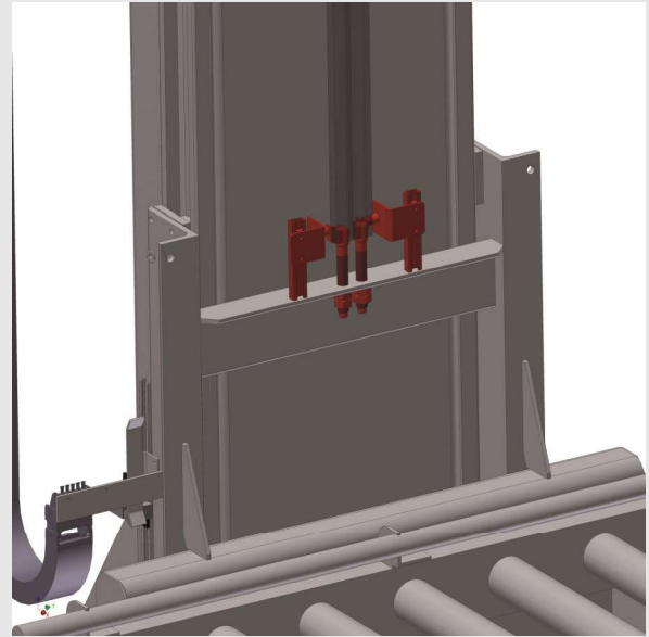
KRC Ketten-/Riemenüberwachung KRC chain-/ belt control
