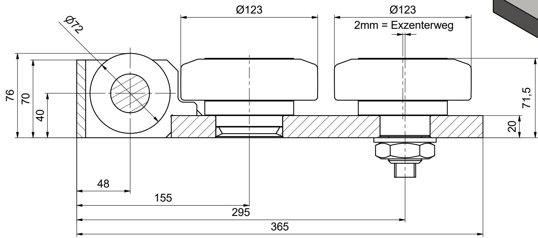
A-A (1:2)
