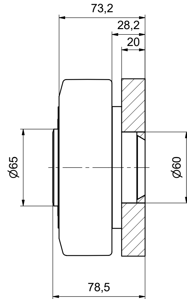
A-A ( 1 : 2 )
